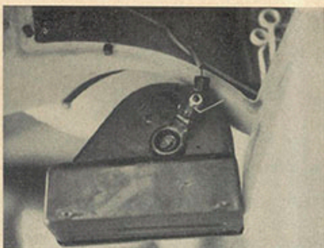
Beim Abnehmen des Luftfilters ist unbedingt darauf zu achten, daß der Bowdenzug vom Starterhebel nicht aus seiner Befestigungsschelle herausrutscht. Wenn es doch passiert, muß unbedingt vor dem Einbau des Luftfilters die Schelle gelöst und der Bowdenzug wieder eingeführt werden.
