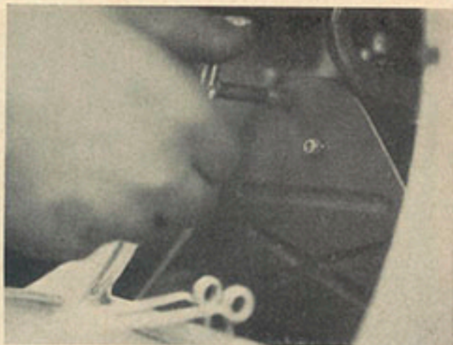
Um überhaupt an den Vergaser heranzukommen, muß erst einmal das Luftfilter abgebaut werden. Das dazu notwendige Lösen der Befestigungsmuttern bereitet keine Schwierigkeiten.
