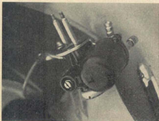
Unten am Vergaser befindet sich eine Muttermutter, nach deren Lösen die Hauptdüse freiliegt.
