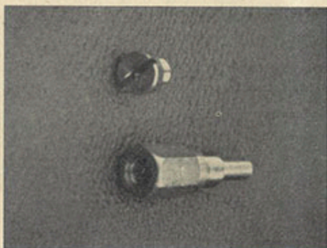
Die Düse selbst ist im Düsenstock festgeschraubt. Im Bilde sind beide Teile auseinander geschraubt zu sehen.
