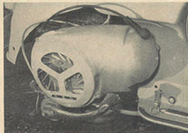
Der gebläsegekühlte 150-ccm-Einzyylinder-Zweitakt-Motor wurde unverändert vom vorherigen Modell übernommen.
